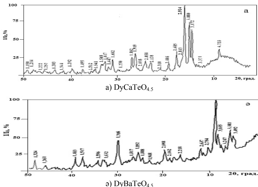
1-сурет. Синтезделген теллуриттердің рентгенограммалары
